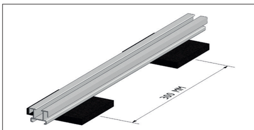
Balk laag 35 x 23 mm op hart afstand 300 mm
