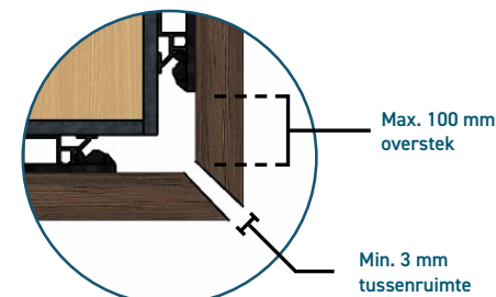
Tussenruimte hoekoplossingen
