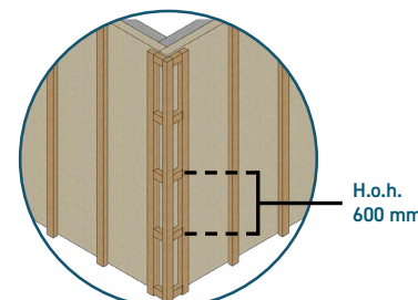
Achterconstructie hoekafwerking
