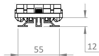
DETAIL A SCHAAL 1 : 3
