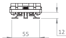
DETAIL A SCHAAL 1 : 3
