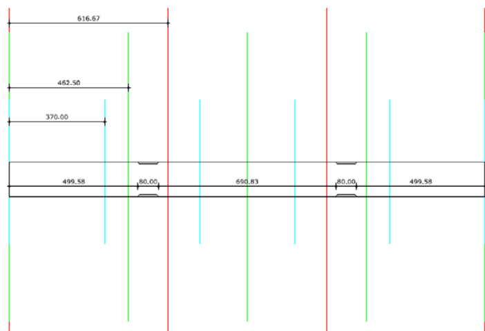
Horizontale gevel (afbeelding 2)
