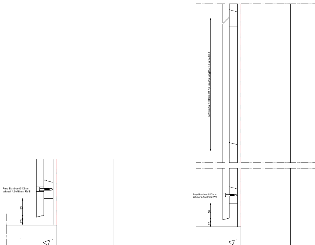
Verticale gevel (afbeelding 3)
