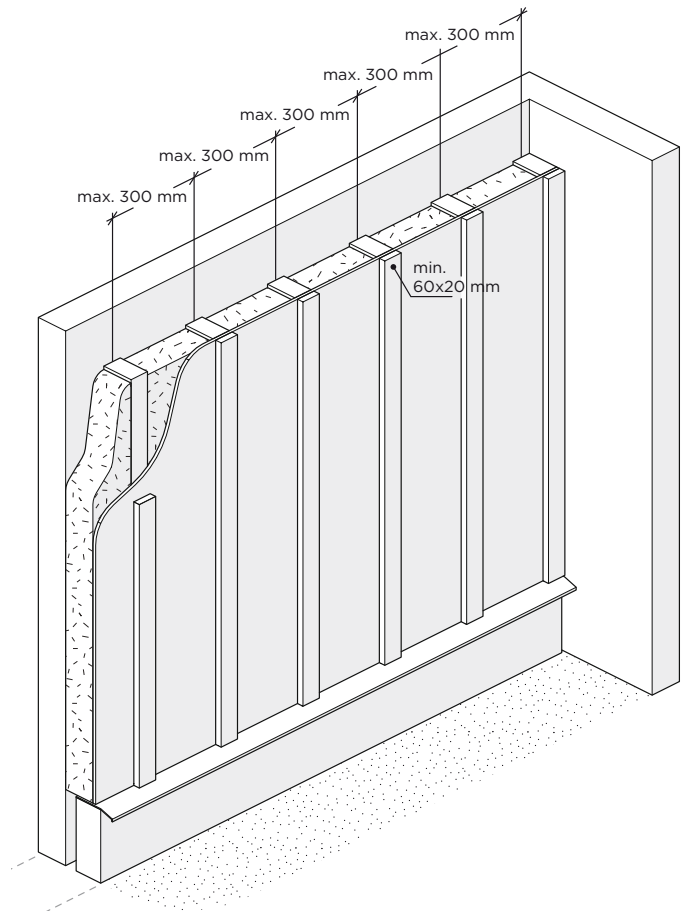
tekening 2 - wildverband
